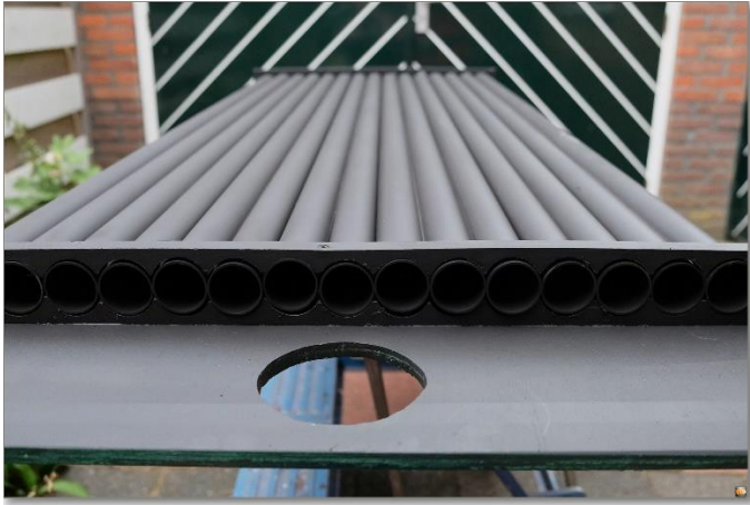
Figuur 4, basis met alu-buizen zonder de omhulling.
